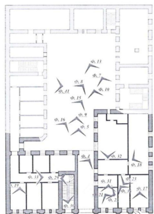
Планы здания, 1 этаж
